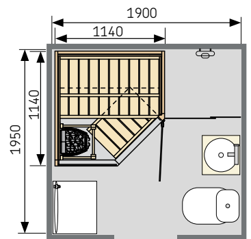
Beispiel für Platzierung der Sirius SC1111K im Badezimmer
