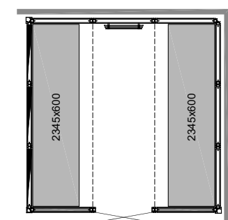
PANACEA 2525 2B Abmessungen: 2525 x 2525 x 2090 mm
