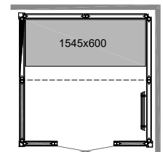
PANACEA 1717 1B Abmessungen: 1725 x 1725 x 2090 mm
